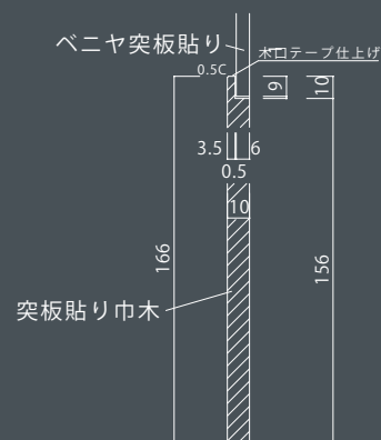
巾木詳細
