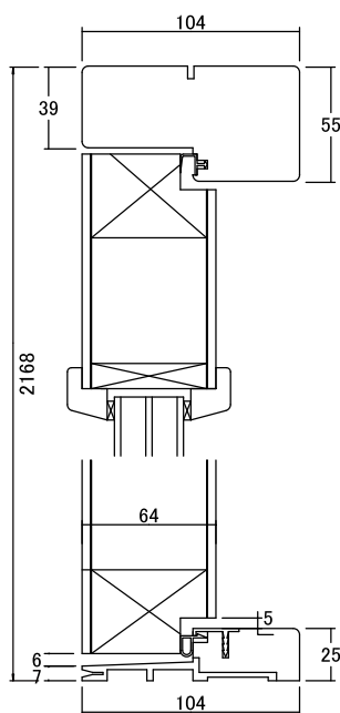
縦断面図 1 : 4
