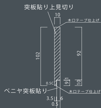
上見切り詳細
