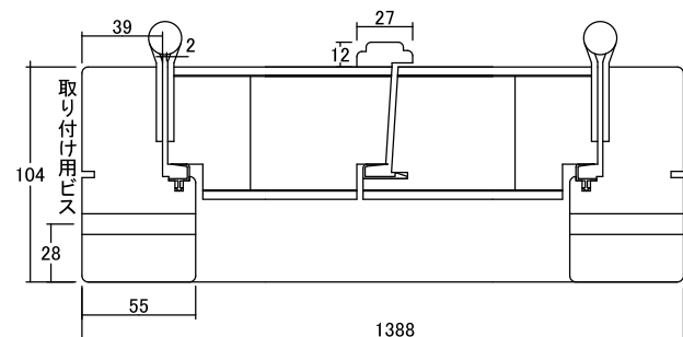
横断面図 1 : 4
