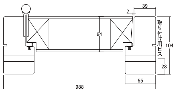
横断面図 1 : 4
