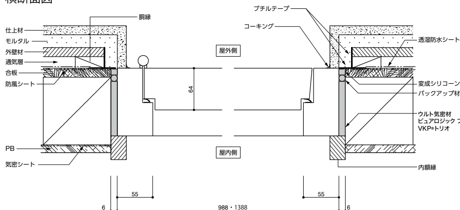
横断面図
