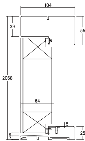
縦断面図 1 : 4
