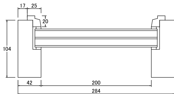
横断面図 1 : 4
