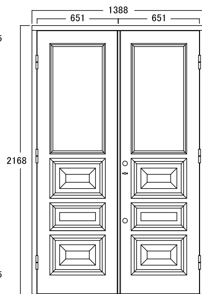
立面図 1 : 30
