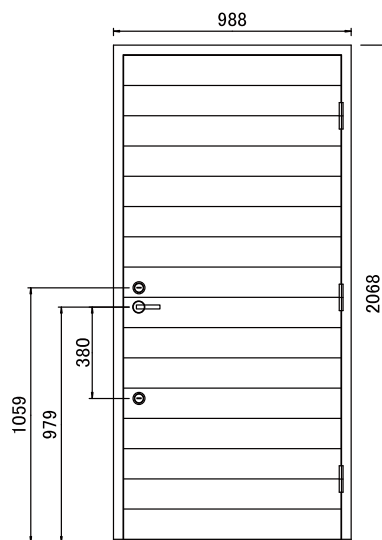
立面図 1 : 30
